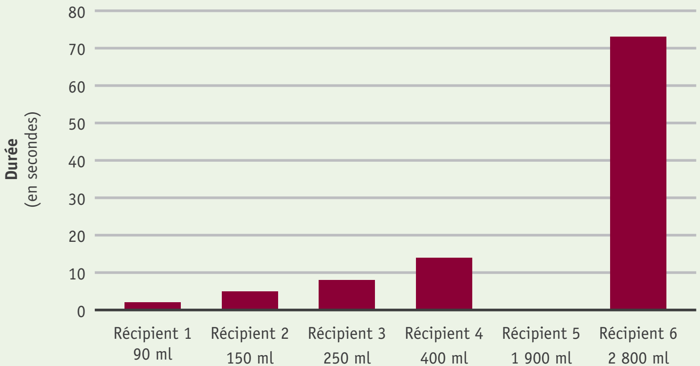
Graphique de la durée de combustion en fonction du volume du récipient
